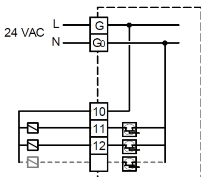
Питание контроллера 24 В переменного тока. Реле 24 В переменного тока.
