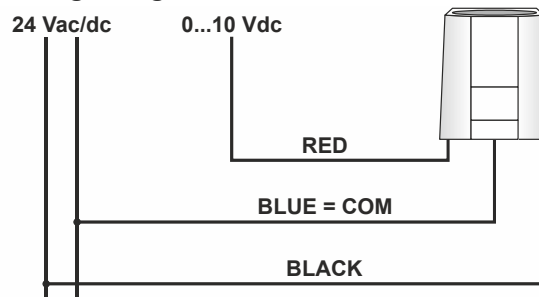
Fig. 7. Wiring diagram
