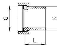
Фитинг резьбовой
